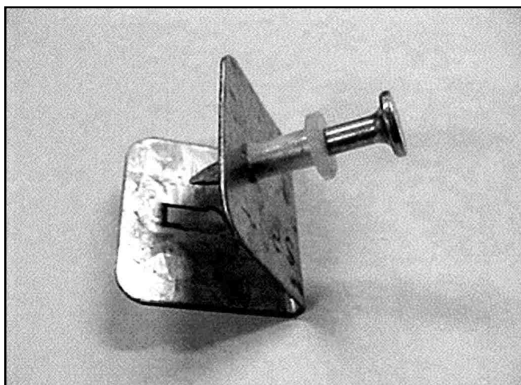
Rys. 5. Klips i kółek do mocowania siatki w podłożu. Klips zakłada się na poprzeczny pręt płaski siatki
